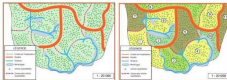
7.2-DES-01 : Exemple de carte de découpage de la zone de coupe en poches 1
